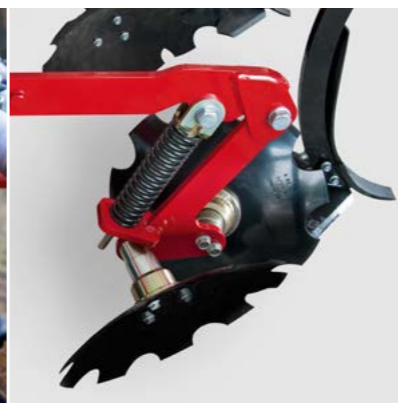
Подпружиненные выравнивающие диски
