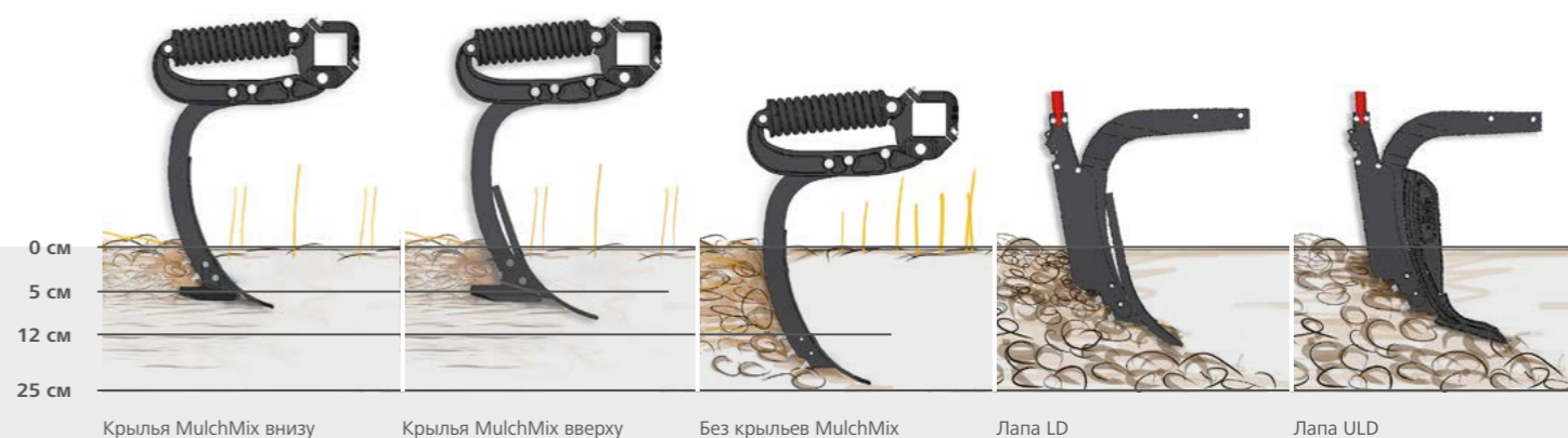
Крылья MulchMix вниз
