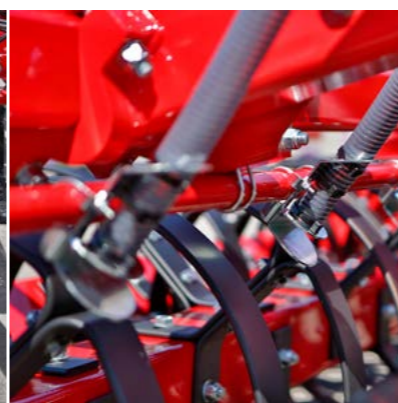
Трубчатые сошники системы MiniDrill расположены перед катком.
