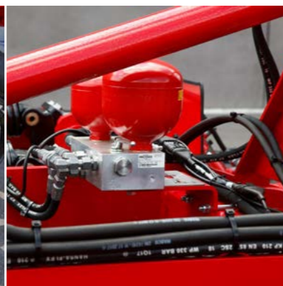
Усилитель тяговой силы – серийно
